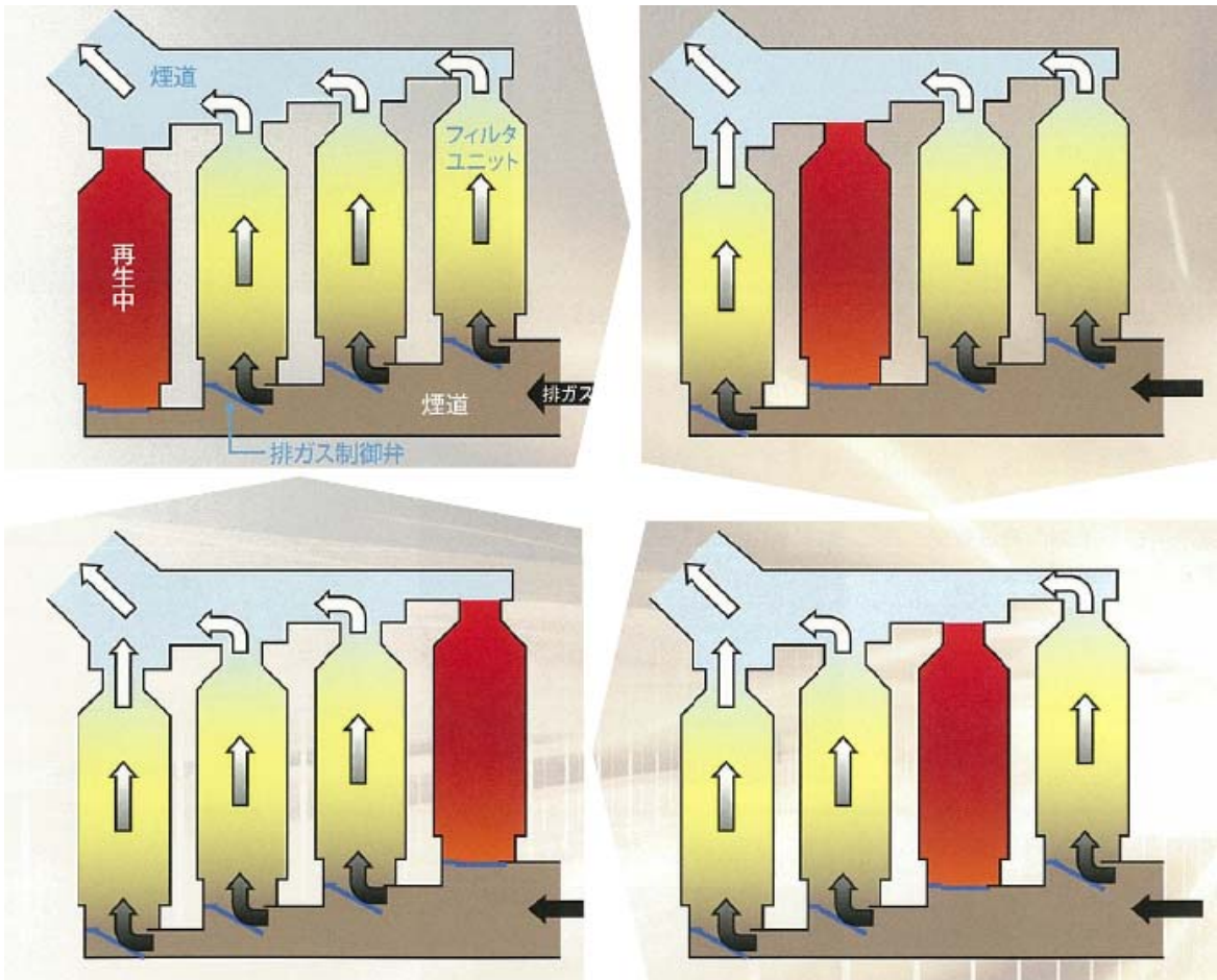
4本の筒状フィルタにて順次再生している
